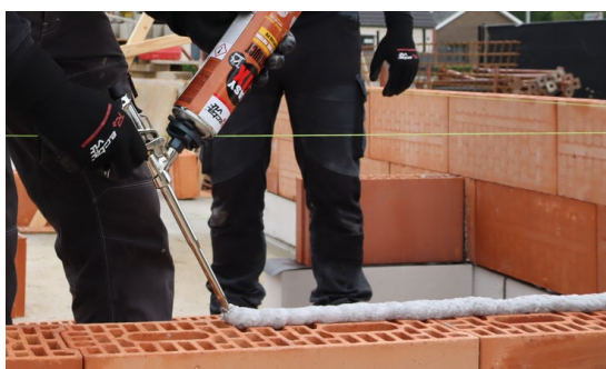
Figuur 1: aanbrengen van de lijm
